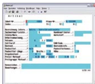
ASCII-Oberfläche
